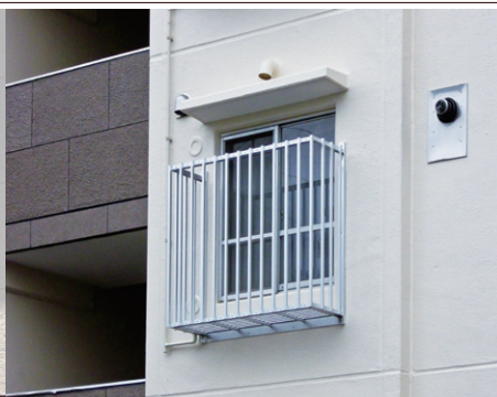
【格子□ -20X20】 縦格子として使用。公共住宅改修工事。
