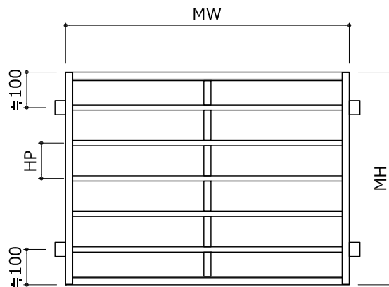
中棧 (MW≥1301) 姿図 S/1:15
