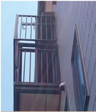
■ 木造住宅 ベランダ手摺の上に取り付 枠：1型 50角柱を手摺で固定し、ブラケットを使用
