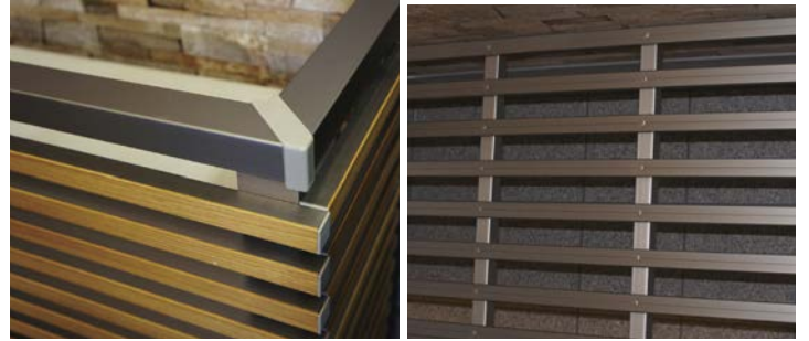
コーナー部上部は、保護樹脂付き。底部は、格子をスノコ状に組付け。
