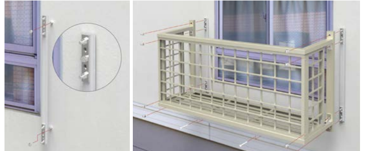
取付材を躯体に固定。
