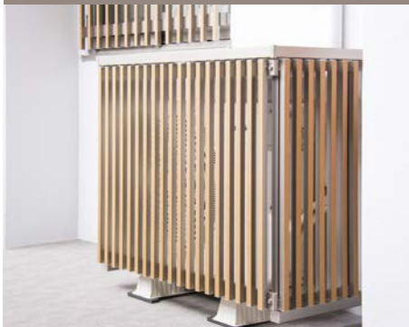
【格子□ -20X20】 木目ラッピング材を使用。底なしで、天板に物を置くことが可能です。共用廊下の室外機カバーとして使用。(オーダータイプ)。
